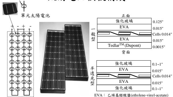
太陽電池模板接線例 太陽電池模板外觀例 太陽電池模板結構例
