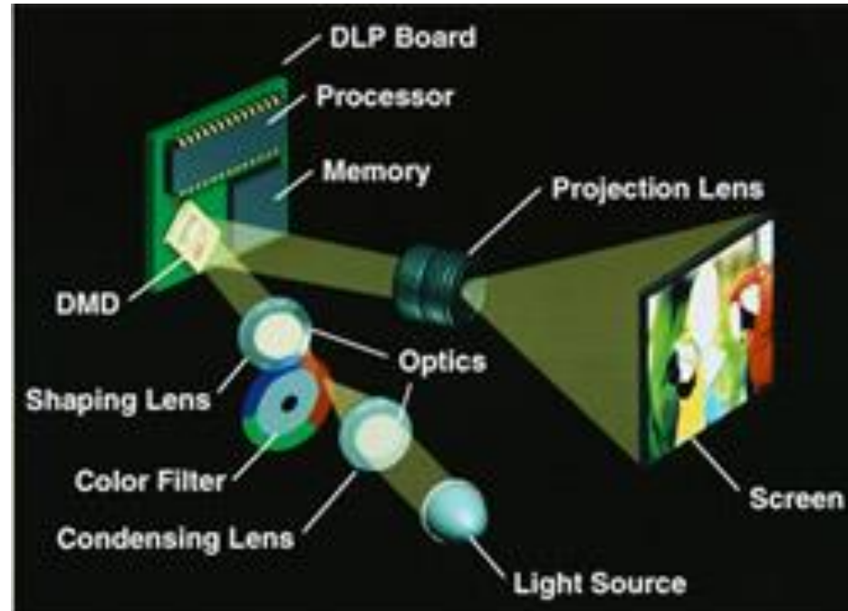
1 DMD
