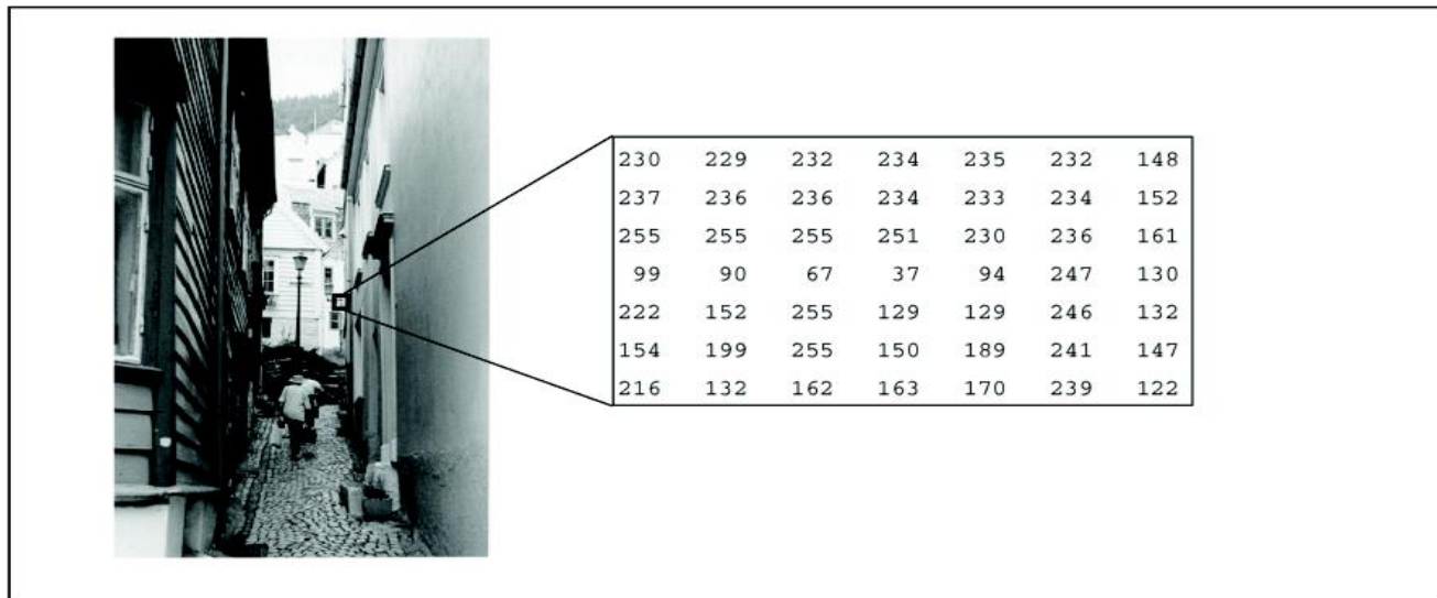
圖 1.17 灰階影像
