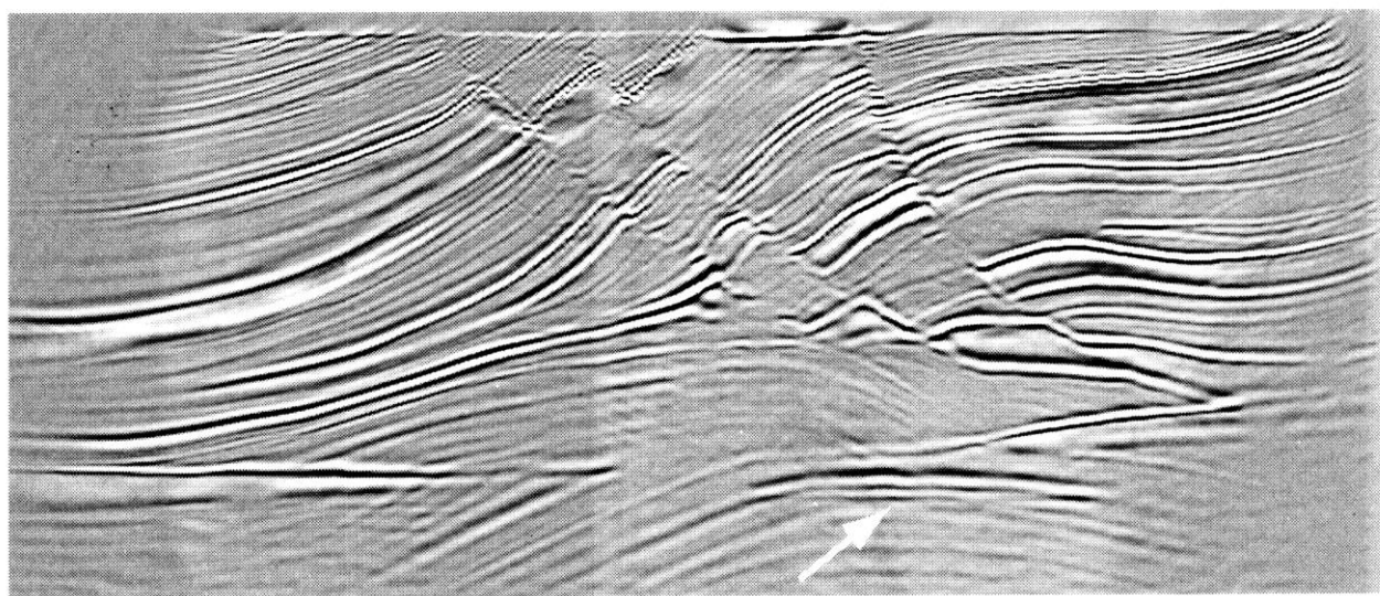
圖 1.19 地震模型的剖面 影像。箭頭指向 碳化氫（油及 / 或氣體）火山 岩。（由桑地亞 國家實驗室的 Dr. Curtis Ober 所提 供。）
